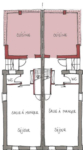
REZ-DE-CHAUSSEE VARIANTE 2
