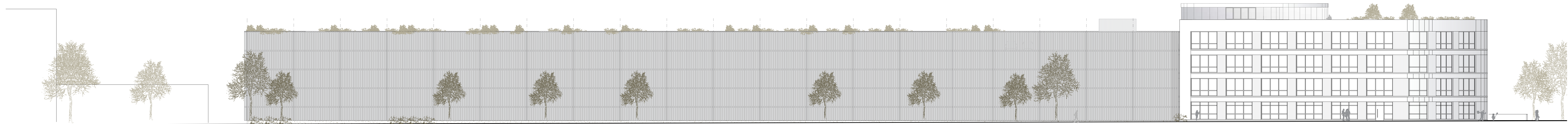
RÜCKANSICHT_BAHNSEITIG
