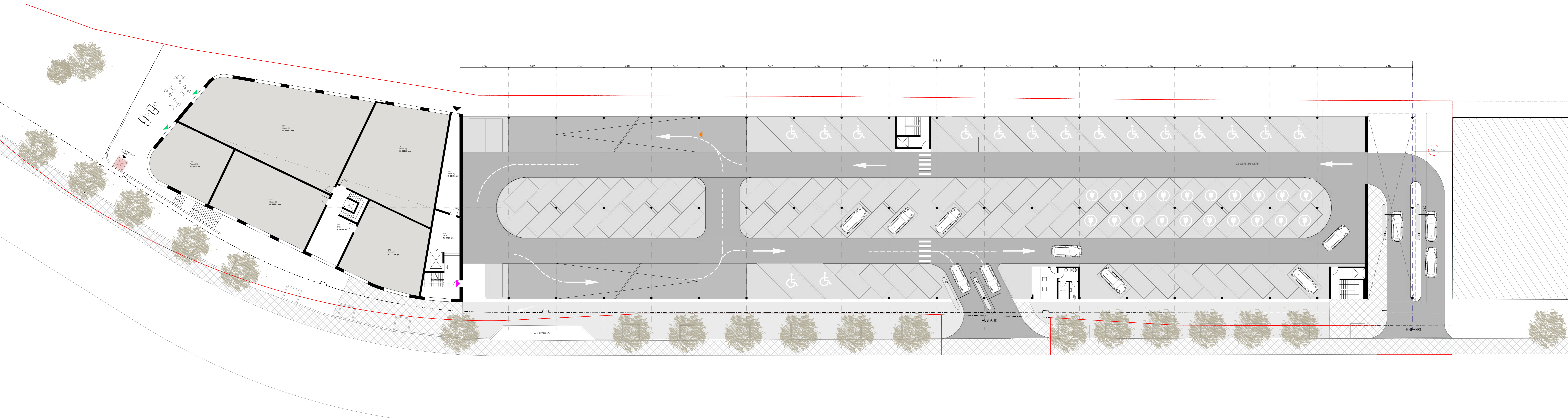
GRUNDRISS ERDGESCHOSS
