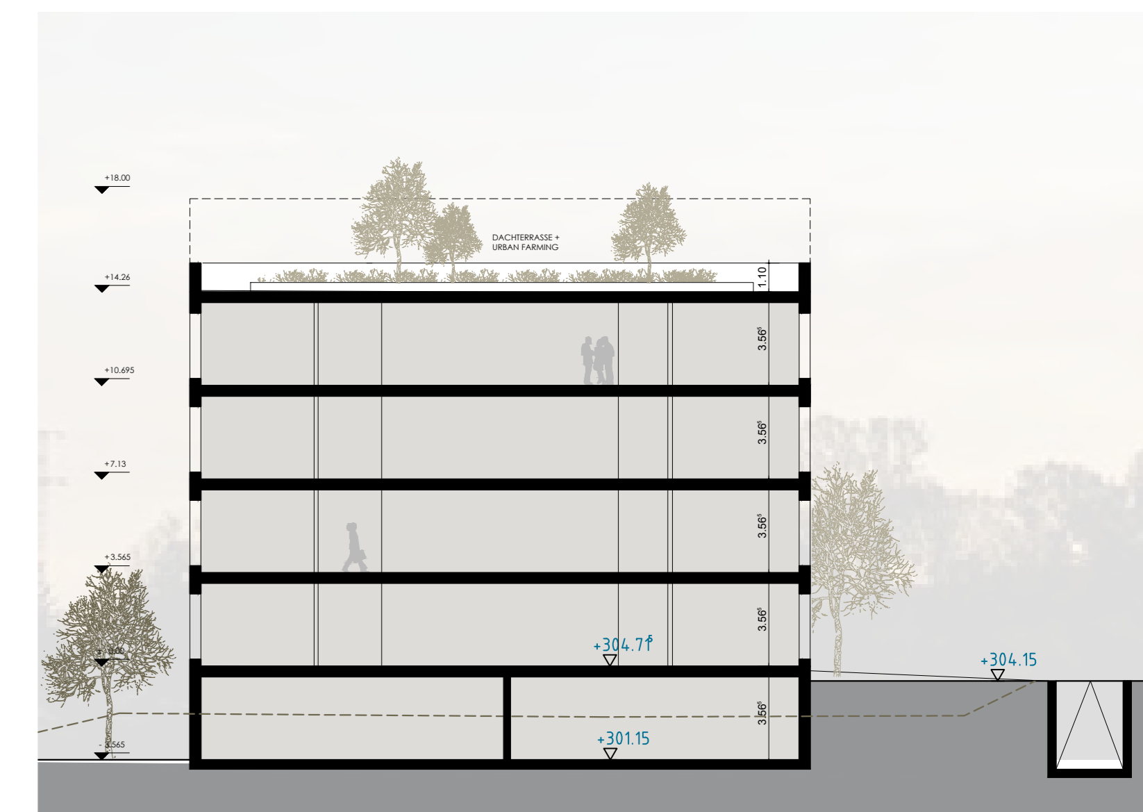
QUERSCHNITT
