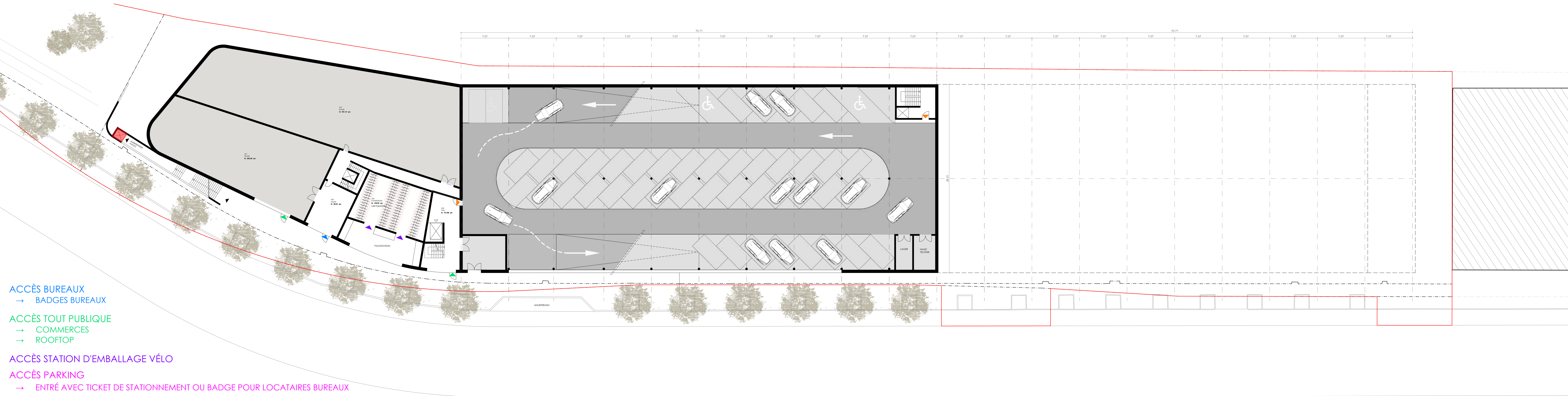
GRUNDRISS UNTERGESCHOSS
