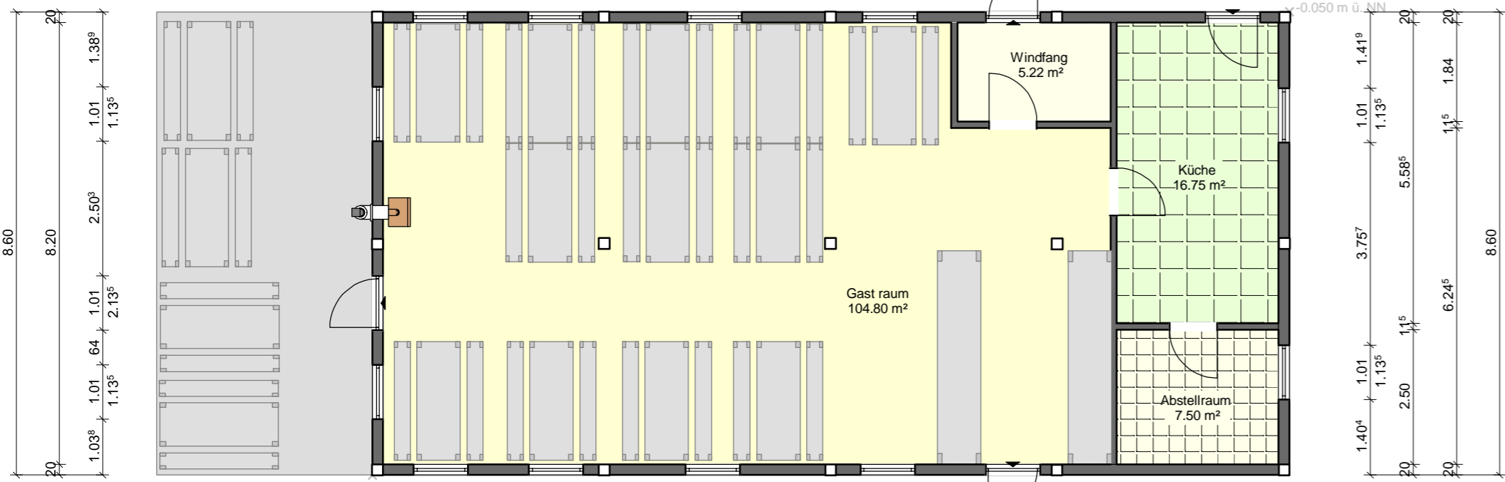
Grundriss
